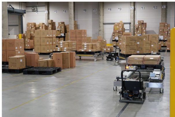
TCセンターに導入している搬送ロボット「キーカート」
